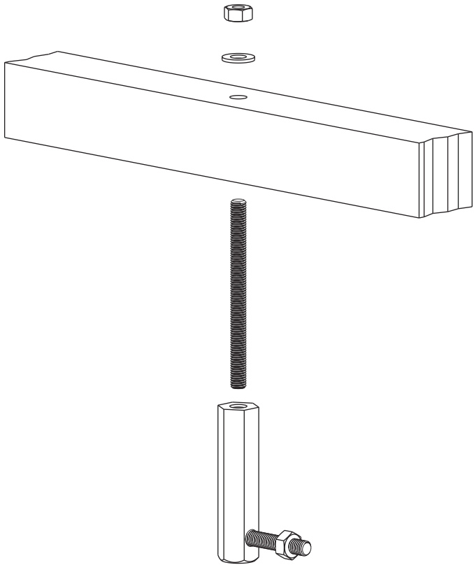
Spiegelbefestigung 2008 Mounting-Kit Variante 1
