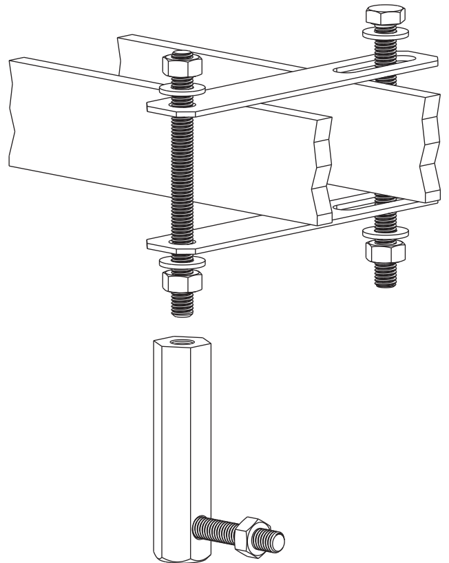
Spiegelbefestigung 2008 Mounting-Kit Variante 2
